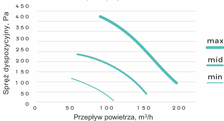
Krzywe wydajności
