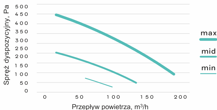
Krzywe wydajności
